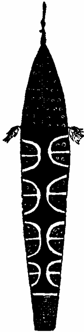
FIG. 38. — Un rombo.
